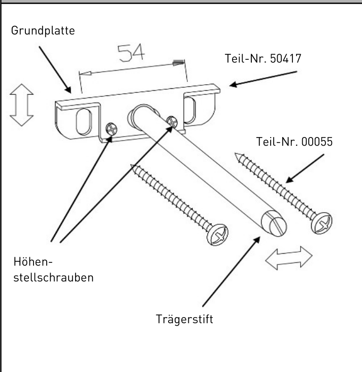
Abbildung 1: Detail Tablarträger
